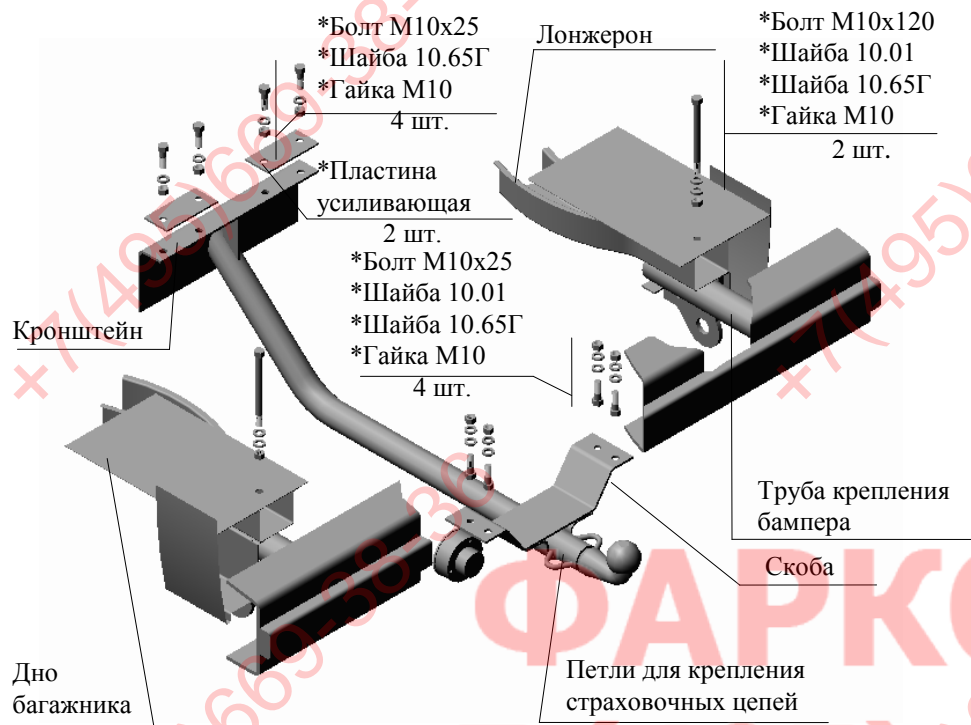
РИС.1 Тягово-сцепное устройство ТСУ 2121 исп.2
